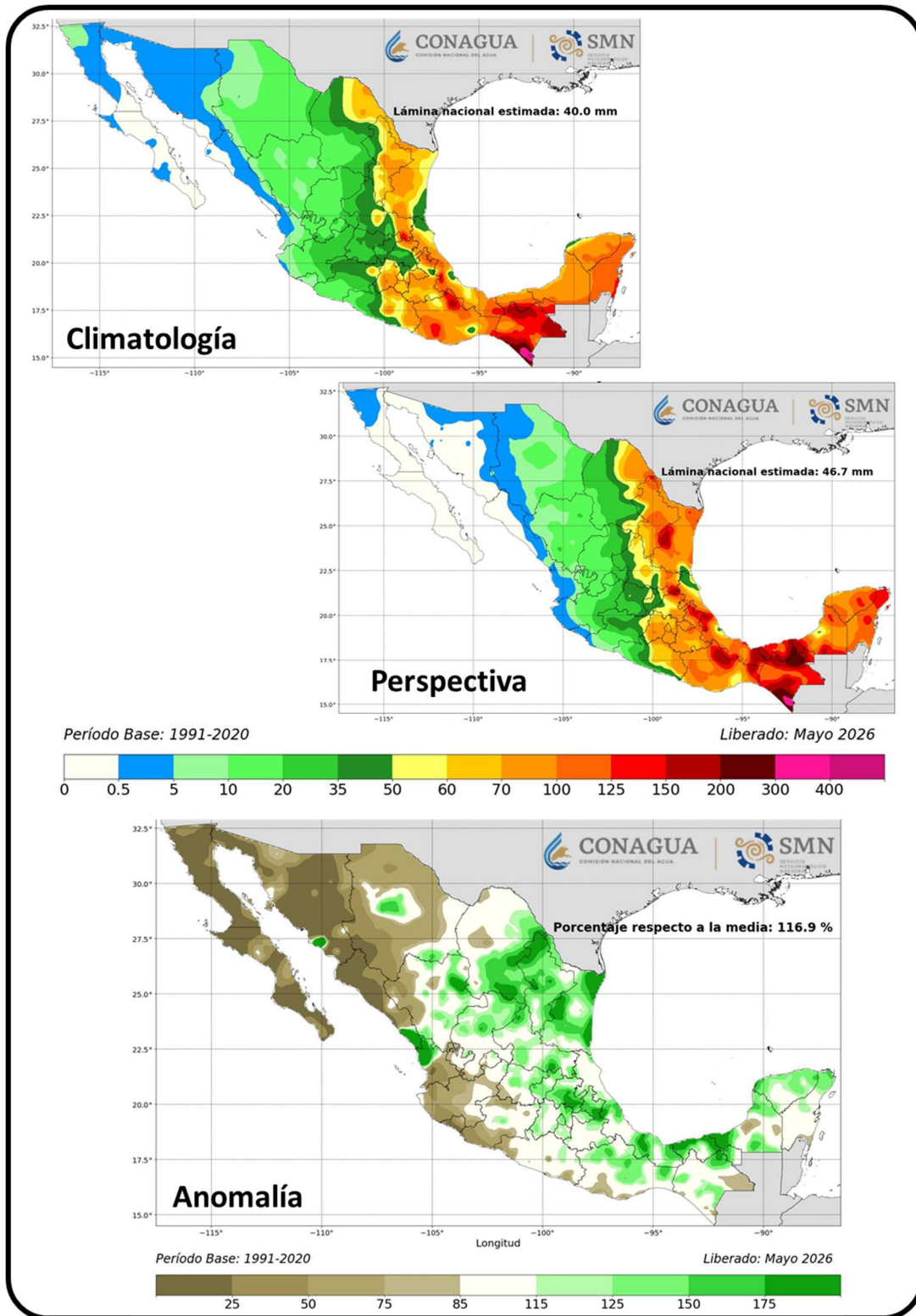
Figura 10. Climatología, Perspectiva y Anomalía de precipitación (mm). Mayo 2026. CONAGUA-SMN.
