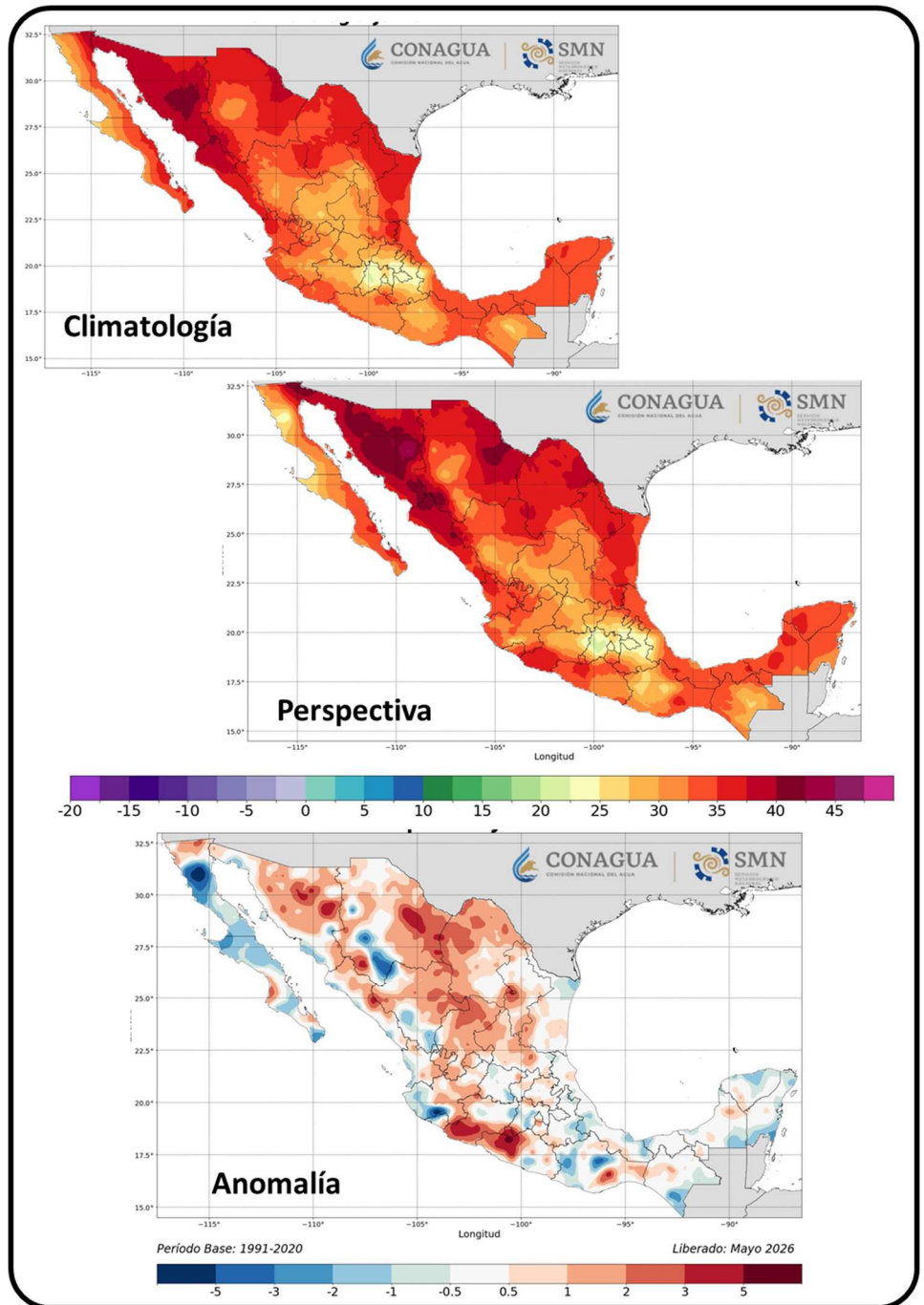
Figura 15. Climatología, Perspectiva y Anomalía de temperatura máxima promedio (°C). Junio de 2026. CONAGUA-SMN.
