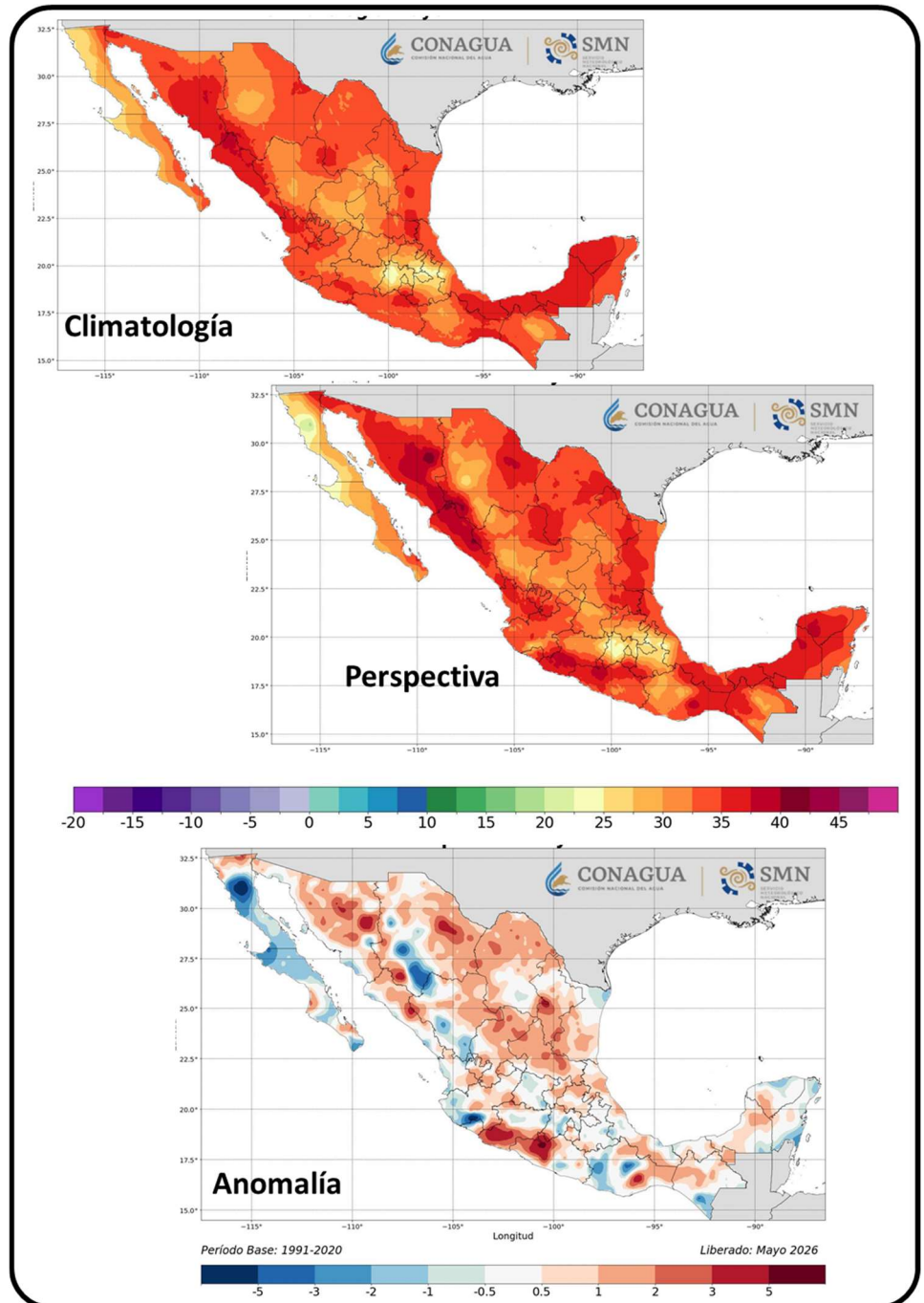
Figura 14. Climatología, Perspectiva y Anomalía de temperatura máxima promedio (°C). Mayo de 2026. CONAGUA-SMN.
