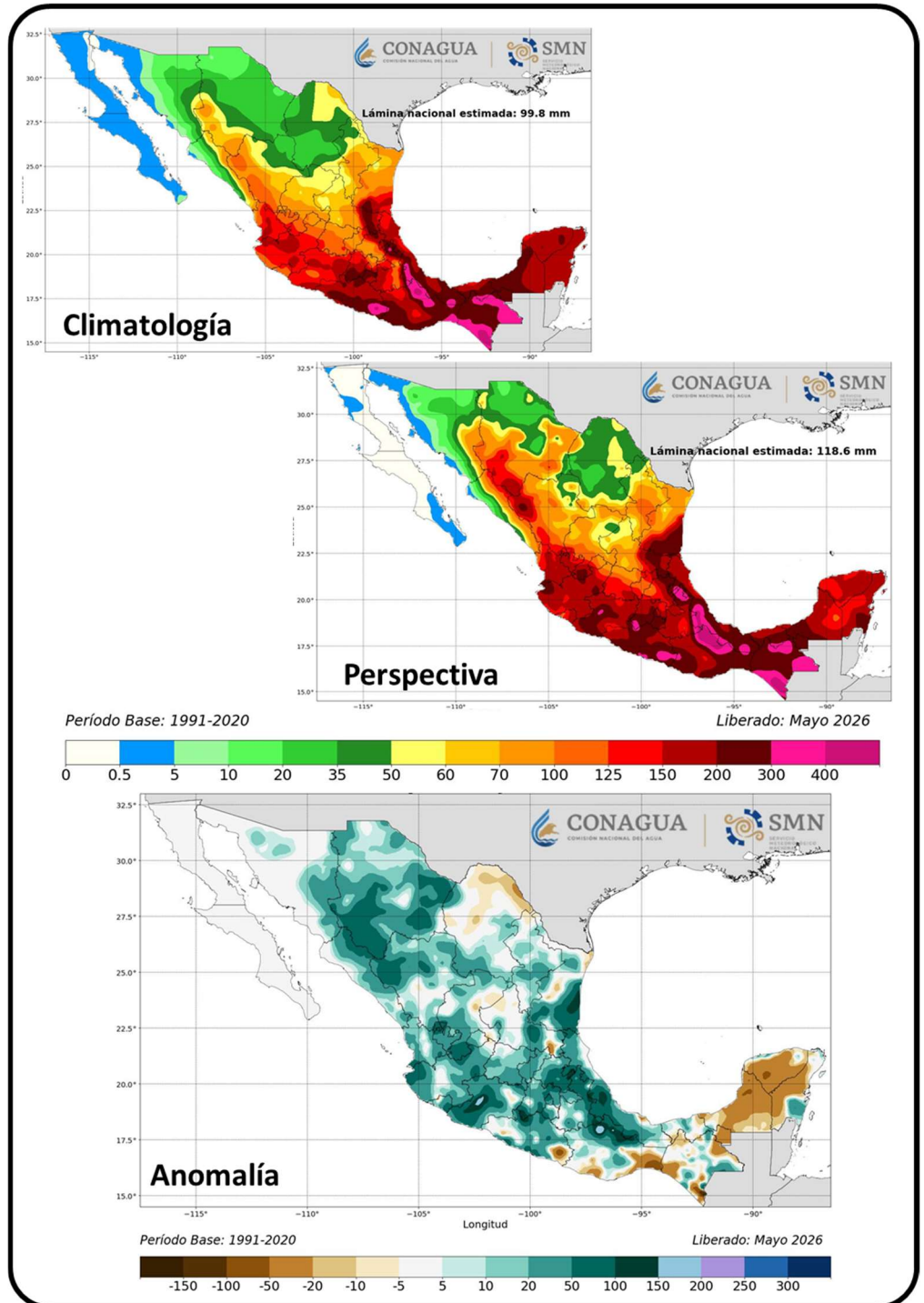
Figura 11. Climatología, Perspectiva y Anomalía de precipitación (mm). Junio 2026. CONAGUA-SMN.
