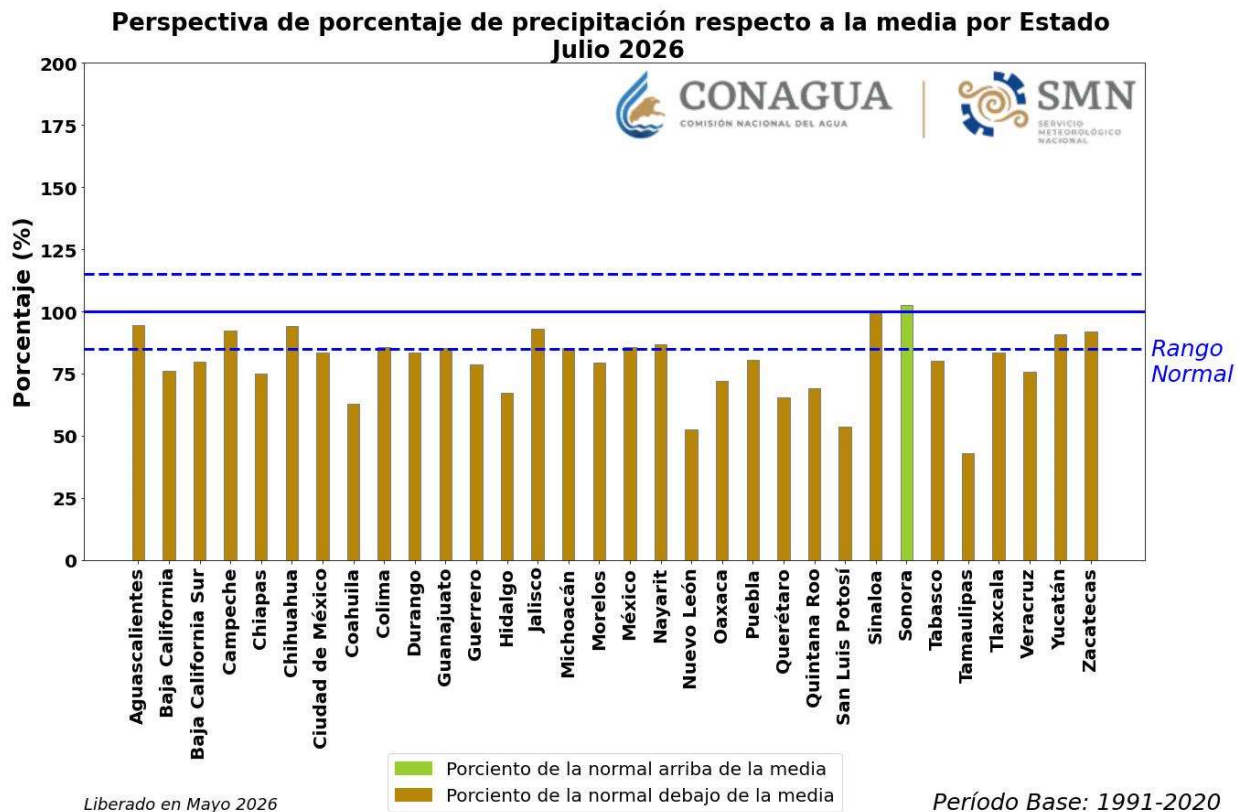
Figura 13. Anomalía de precipitación (mm). Julio 2026. CONAGUA-SMN.
