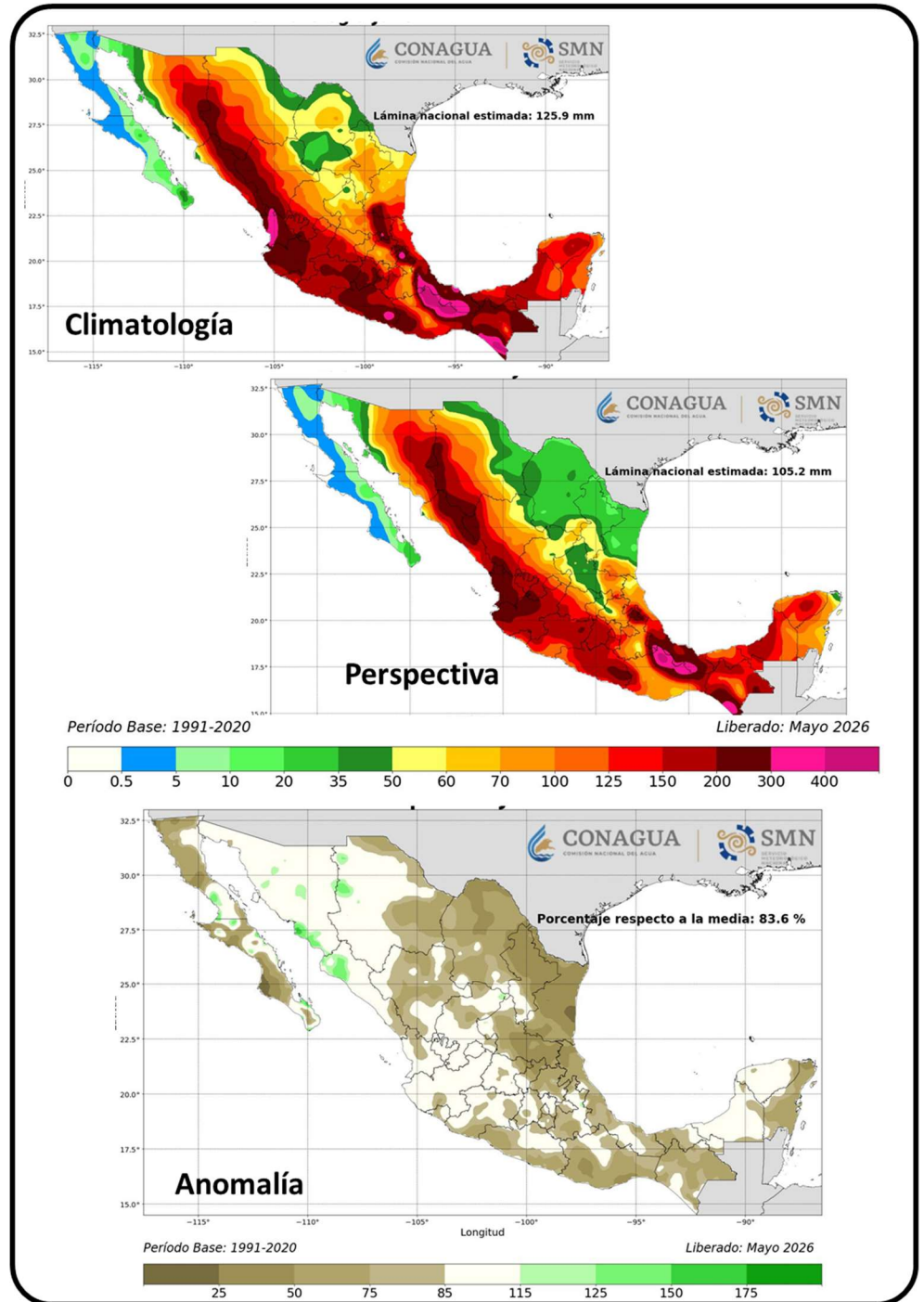
Figura 12. Climatología, Perspectiva y Anomalía de precipitación (mm). Julio 2026. CONAGUA-SMN.
