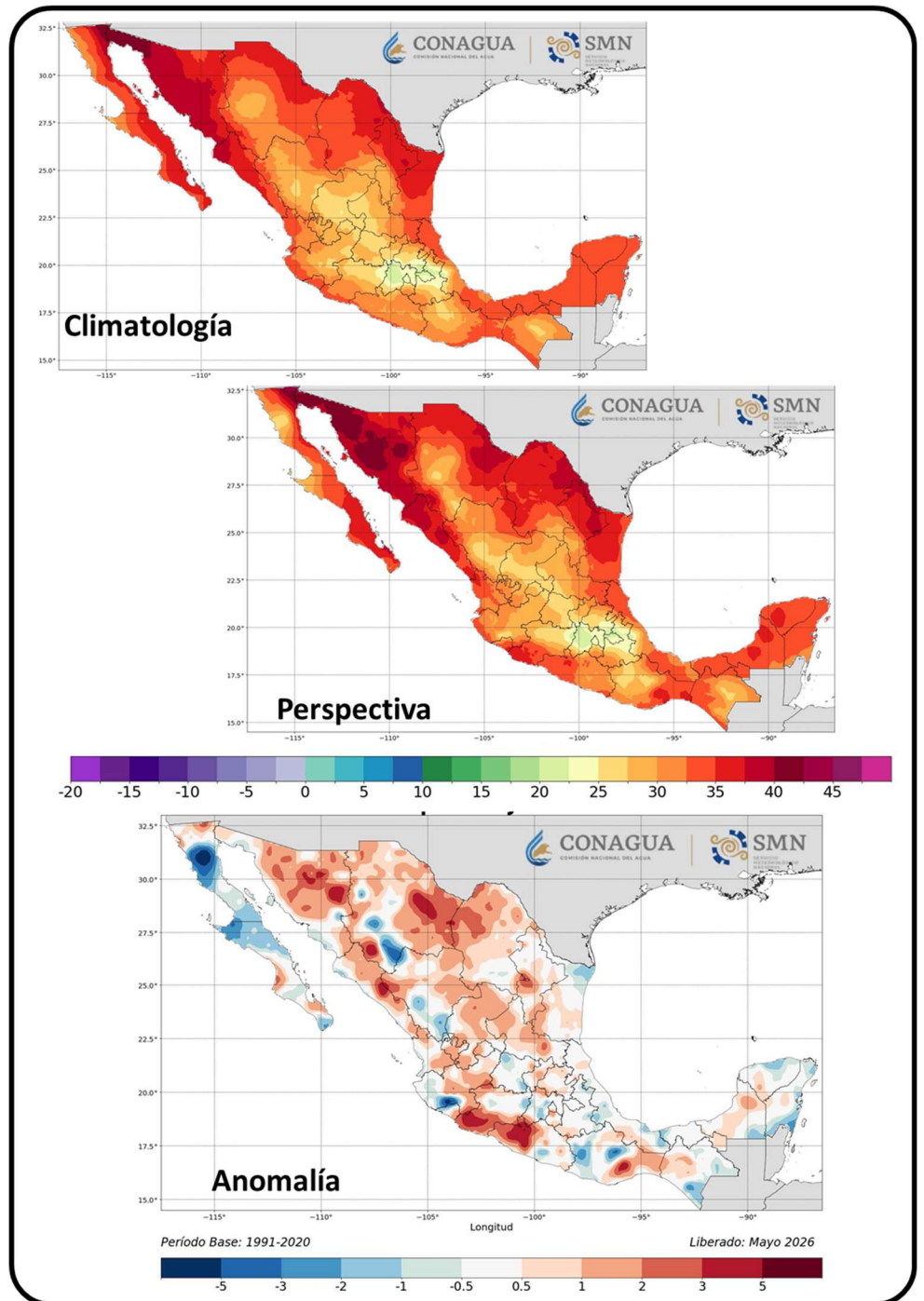
Figura 16. Climatología, Perspectiva y Anomalía de temperatura máxima promedio (°C). Julio de 2026. CONAGUA-SMN.
