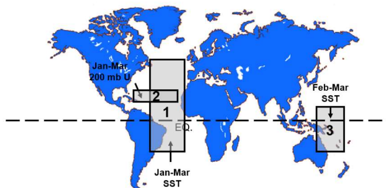
Figura 19. Zonas de formación de Ciclones Tropicales en el Atlántico.
